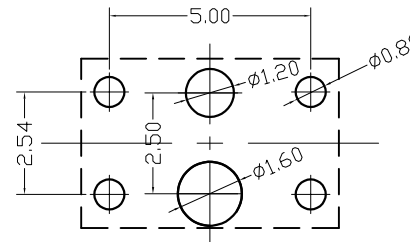
PCB-LAYOUT 尺寸公差: ±0.1
